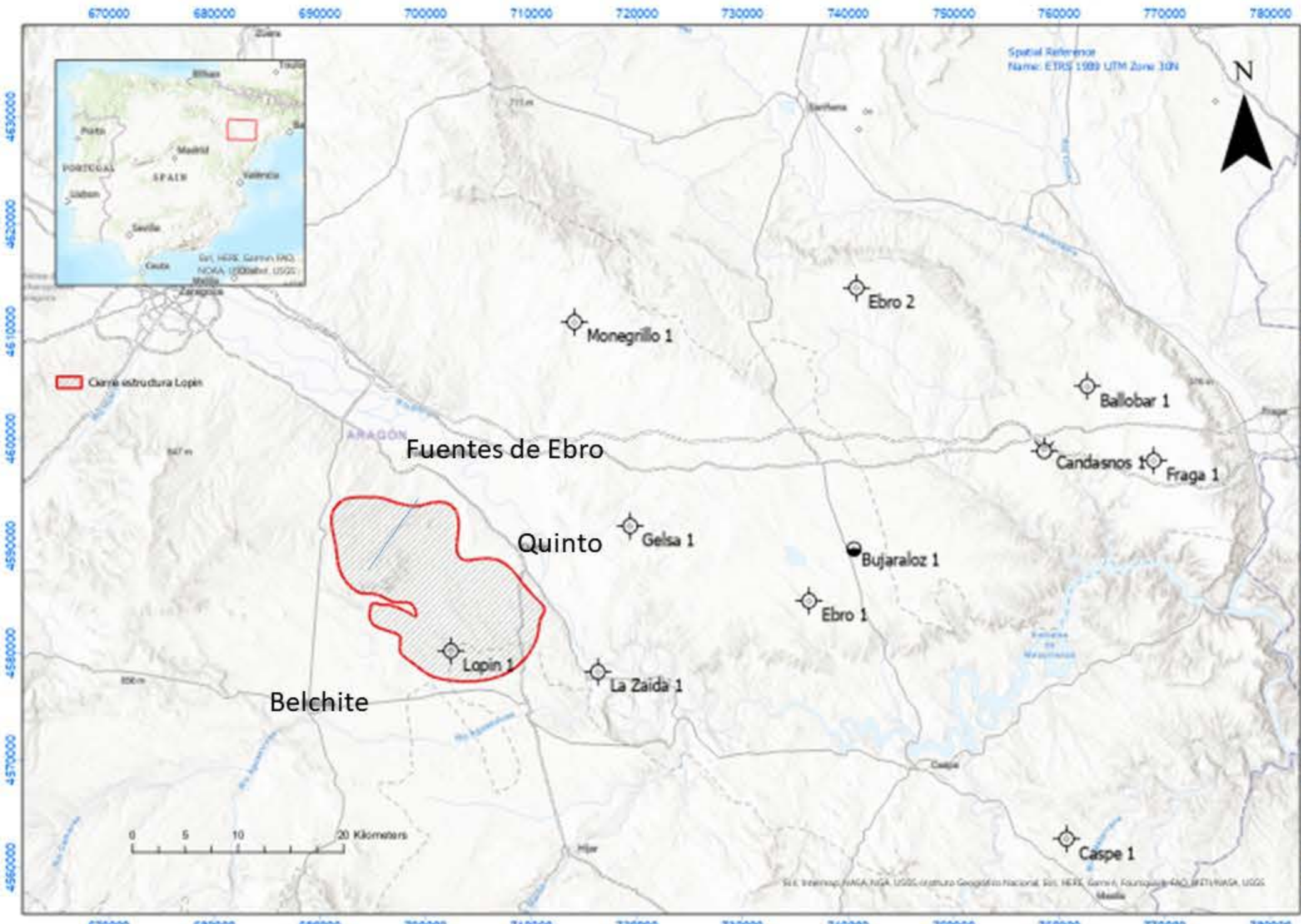
Situación de antiguos pozos de exploración petrolera de la zona (1950-1980)
