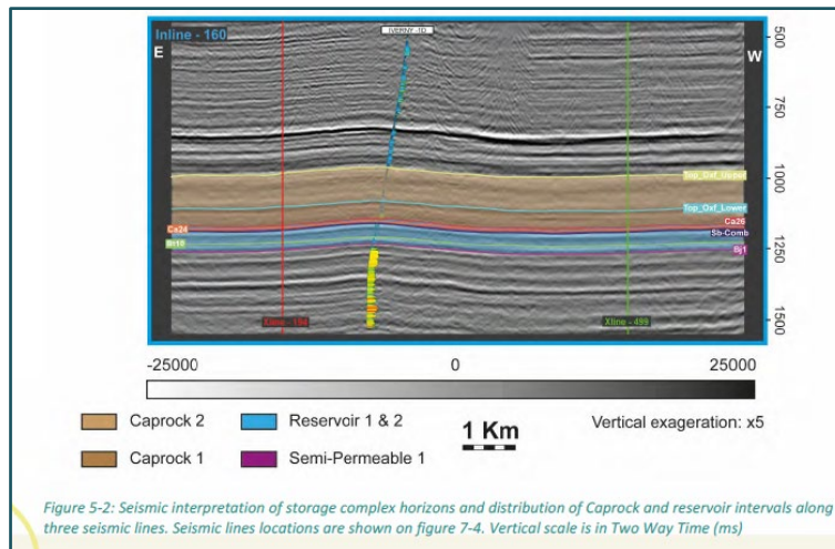
Figure 2. Représentation du sous-sol à Grandpuits, France, obtenue par interprétation sismique. Tirée du livrable PilotSTRATEGY D2.7 8
