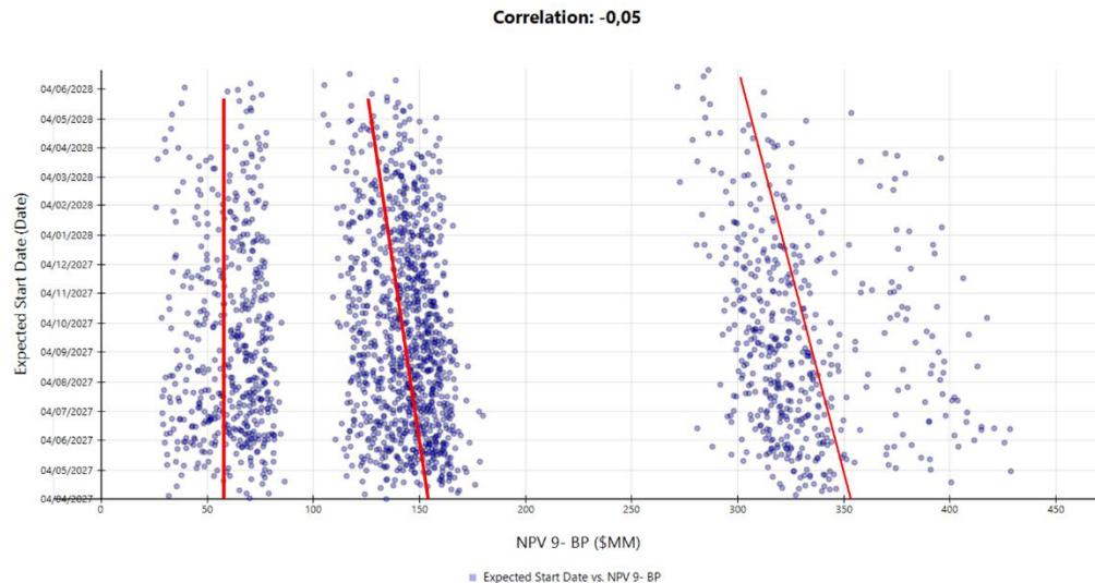
Figura 5.17: Impacto en el retraso en la obtención de permisos sobre el NPV (9%, 2025)
